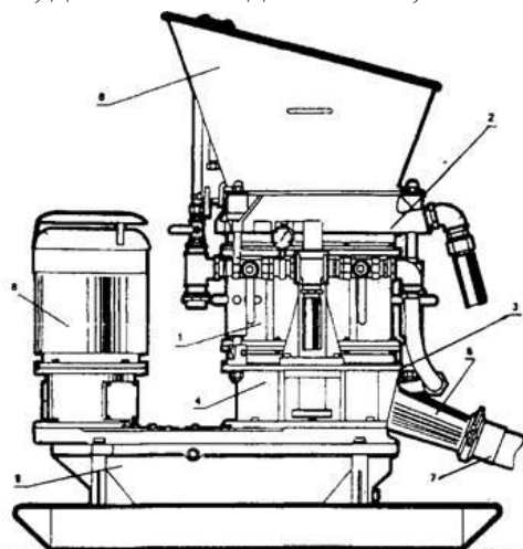
Рис.3.Бетоноукладчик БМ-86: 1-барабан, 2 - неподвижный верхний диск, 3 - неподвижный нижний диск, 4 - основание дозатора, 5 - входной патрубков, 6 - загрузочная воронка, 7 - материальный шланг, 8 - электродвигатель, 8 - редуктор.
