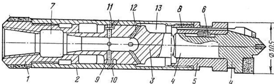
Рис. 2.31. Пневмоударник ПП - 105 – 22
